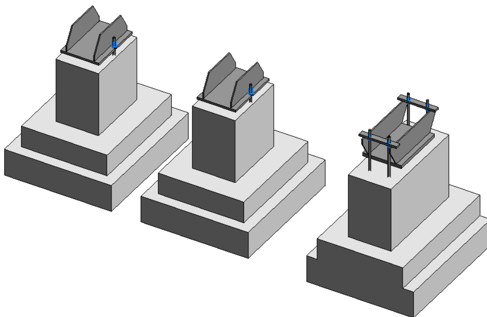
Размеры опорных плит баз колонн
